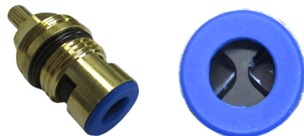
6116070 "VITONE 1/2" 1/4 DI GIRO ACQUA FREDDA ATT. BROCCIA 8x20" / COLD WATER JOINT 8X20"
