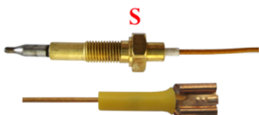
TERMOCOPPIA CON GIUNZIONE CAVI THERMOCOUPLE WITH FASTON CONNECTION
