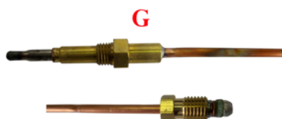
GIUNTO SPECIALE SPECIAL JOINT
