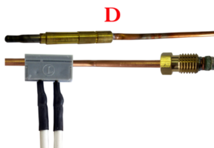
GIUNTO UNIFICATO - INTERROTTA CABLATA UNIFIED SLEEVE - INTERRUPTED CABLED
