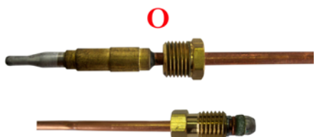
GIUNTO SPECIALE TARGET SPECIAL JOINT TARGET
