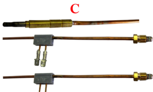
GIUNTO UNIFICATO - INTERROTTA UNIFIED SLEEVE - INTERRUPTED
