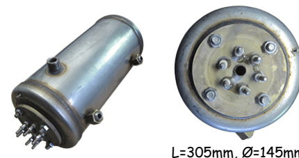
L=305mm, Ø=145mm
